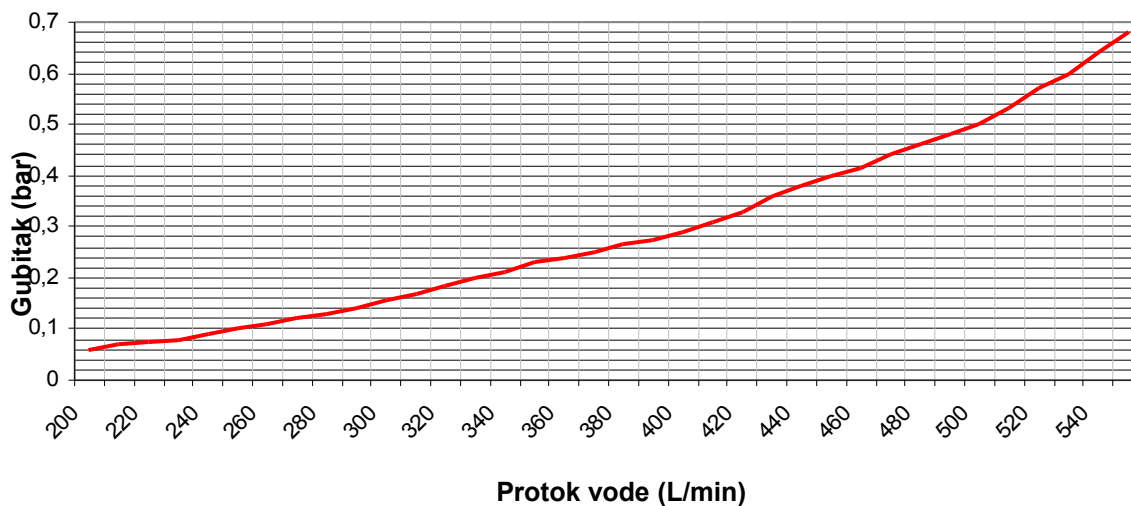
Gubitak tlaka s obzirom na protok vode (ulazni tlak 6 bar)
