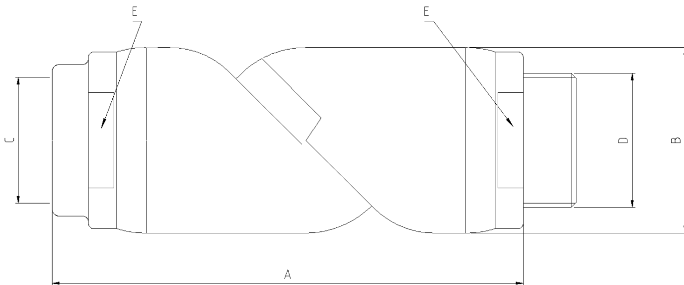
Dijagram (za DV40 spojnicu)
